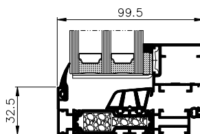
rez štruktúrálnym otváracím oknom
