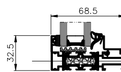
rez fixným oknom
