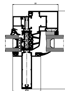
vodorovný rez napojenia otváracého krídla s fixným polom
