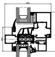
zvislý rez napojenia otváracého krídla s fixným polom
